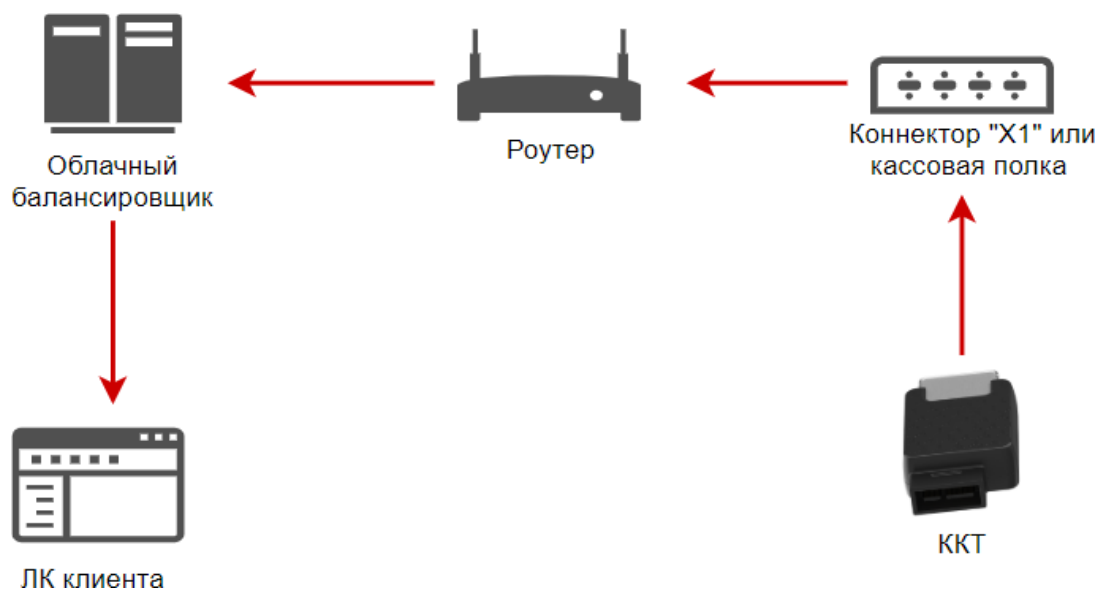
Рисунок 6. Общая схема подключения при использовании «Облачного балансировщика»
